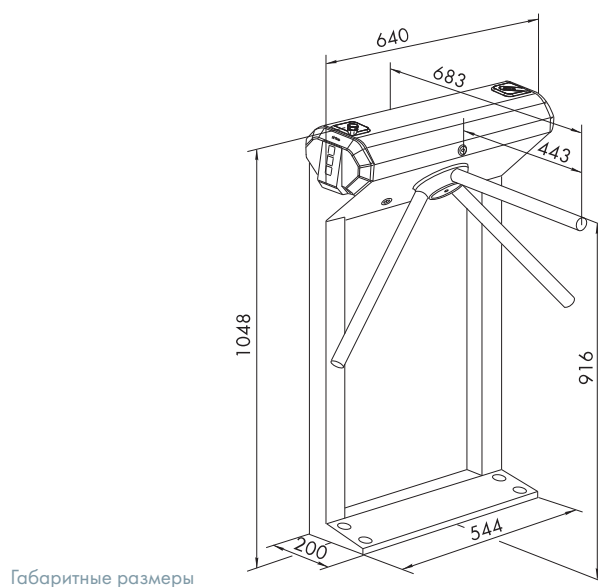
Габаритные размеры
