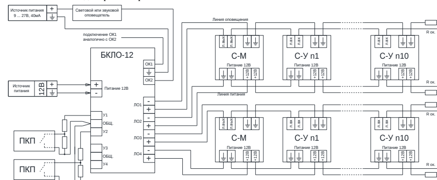
Рисунок – 4 Схема подключения оповещателей по варианту №3 (п. 3.3.2 настоящего руководства по эксплуатации), выходов транзисторных ключей ОК1 «ПИТАНИЕ» и ОК2 «НЕИСПРАВНОСТЬ».
