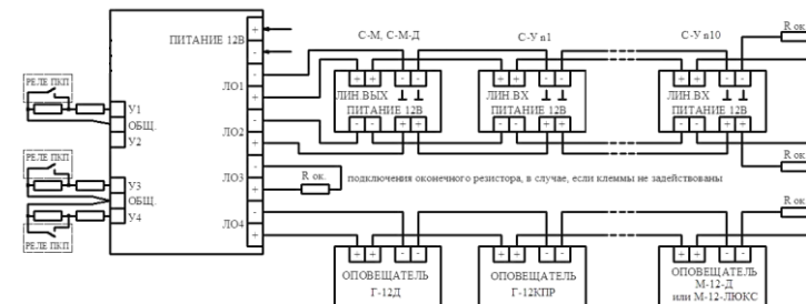
Рисунок – 3 Схема подключения оповещателей по варианту №2 (п. 3.3.1 настоящего руководства по эксплуатации).
