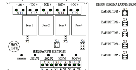
Рисунок-2 Схема подключения БКЛО
