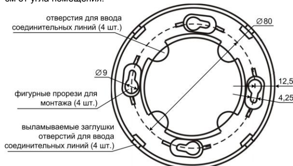
Рис.3 База извещателя. Расположение отверстий для крепления. Присоединительные размеры
