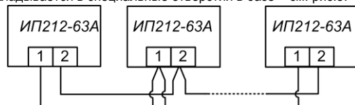
Рис.4 Схема соединения извещателей в группу
