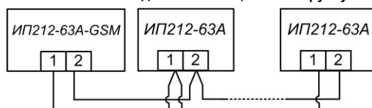
Рис.5 Схема соединения извещателей в группу
