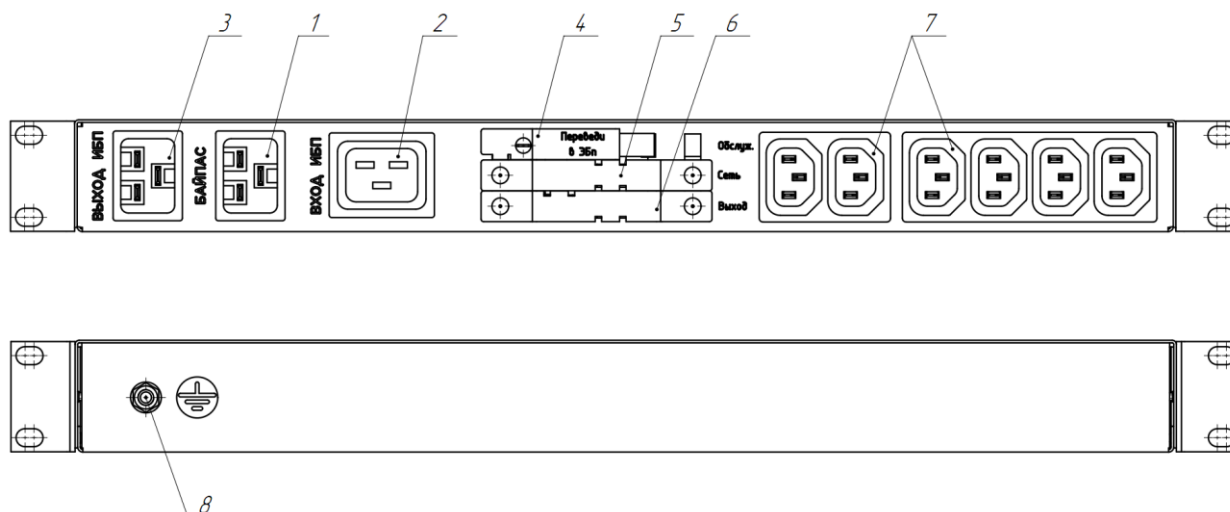
Рис. 2 Расположение разъемов подключения и автоматических выключателей
