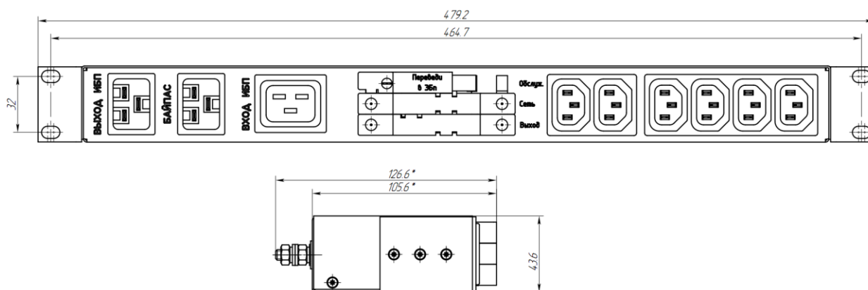
Рис. 1 Габаритно-присоединительные размеры ПР. Вид спереди и сбоку.
