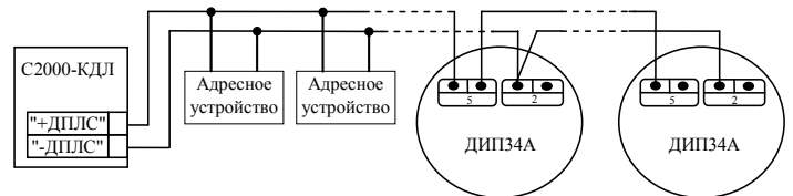
Рисунок 1. Схема соединений
