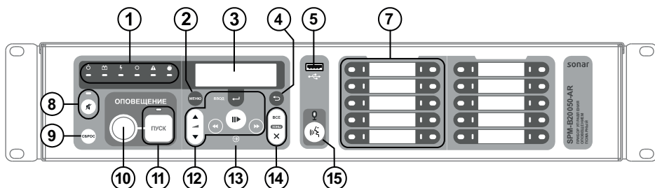
Рисунок 4 – Лицевая панель моделей Sonar SPM-B20xxx-xx (20 зон)
