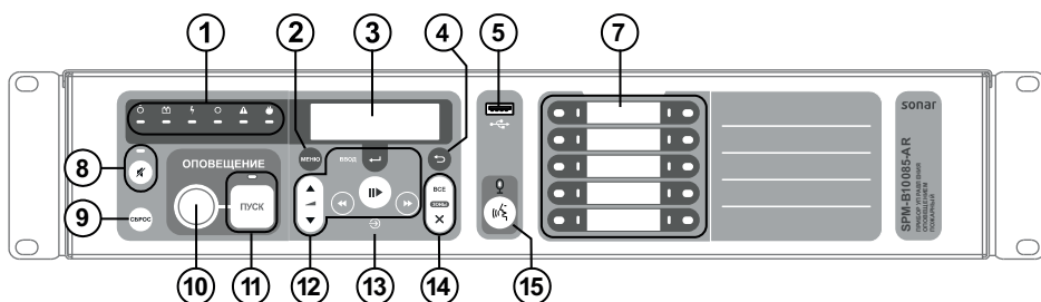
Рисунок 3 – Лицевая панель моделей Sonar SPM-B10xxx-xx (10 зон)
