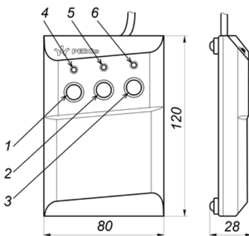
Рисунок 3. Общий вид и габаритные размеры ПДУ
