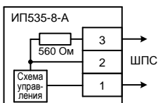
Рис.2 Схема подключения к ШПС ППКП «Кварц» «Карат»
