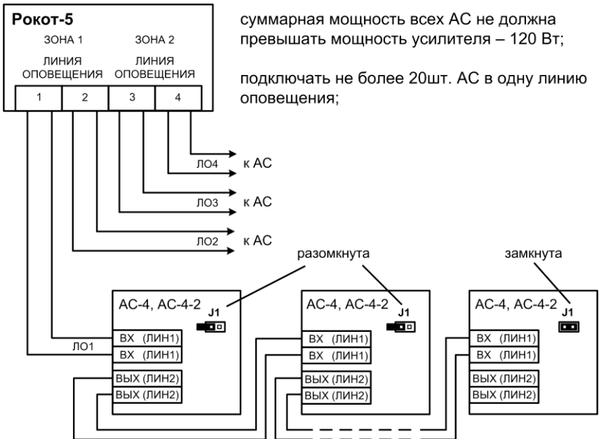
Рис.5а Схема подключения AC-4 и AC-4-2 к линиям оповещения
