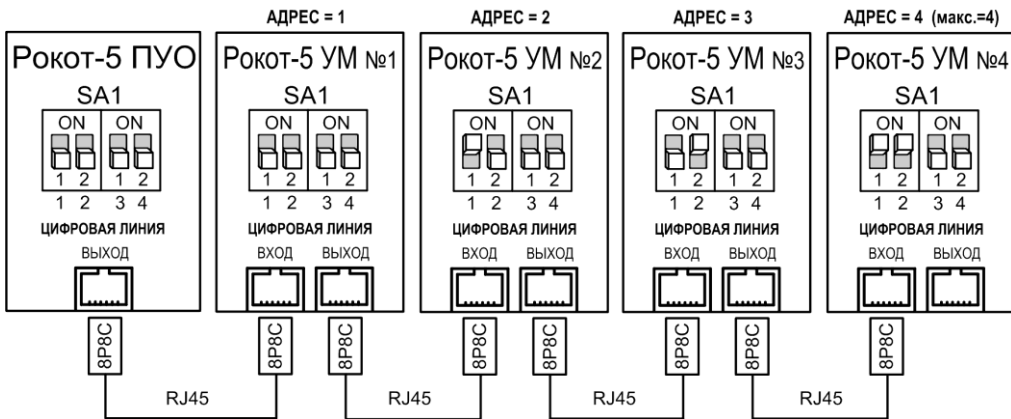
Рис.7 Схема соединения «Рокот-5 ПУО» и «Рокот-5 УМ» (всего можно подключить до 4-х усилителей мощности)
