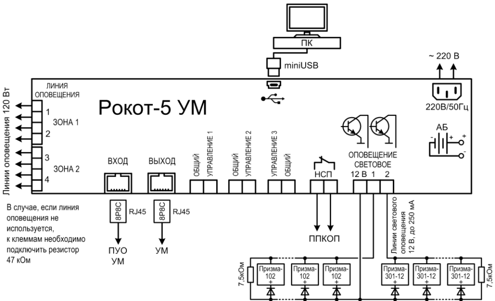
Рис.6 Схема внешних подключений «Рокот-5 УМ»
