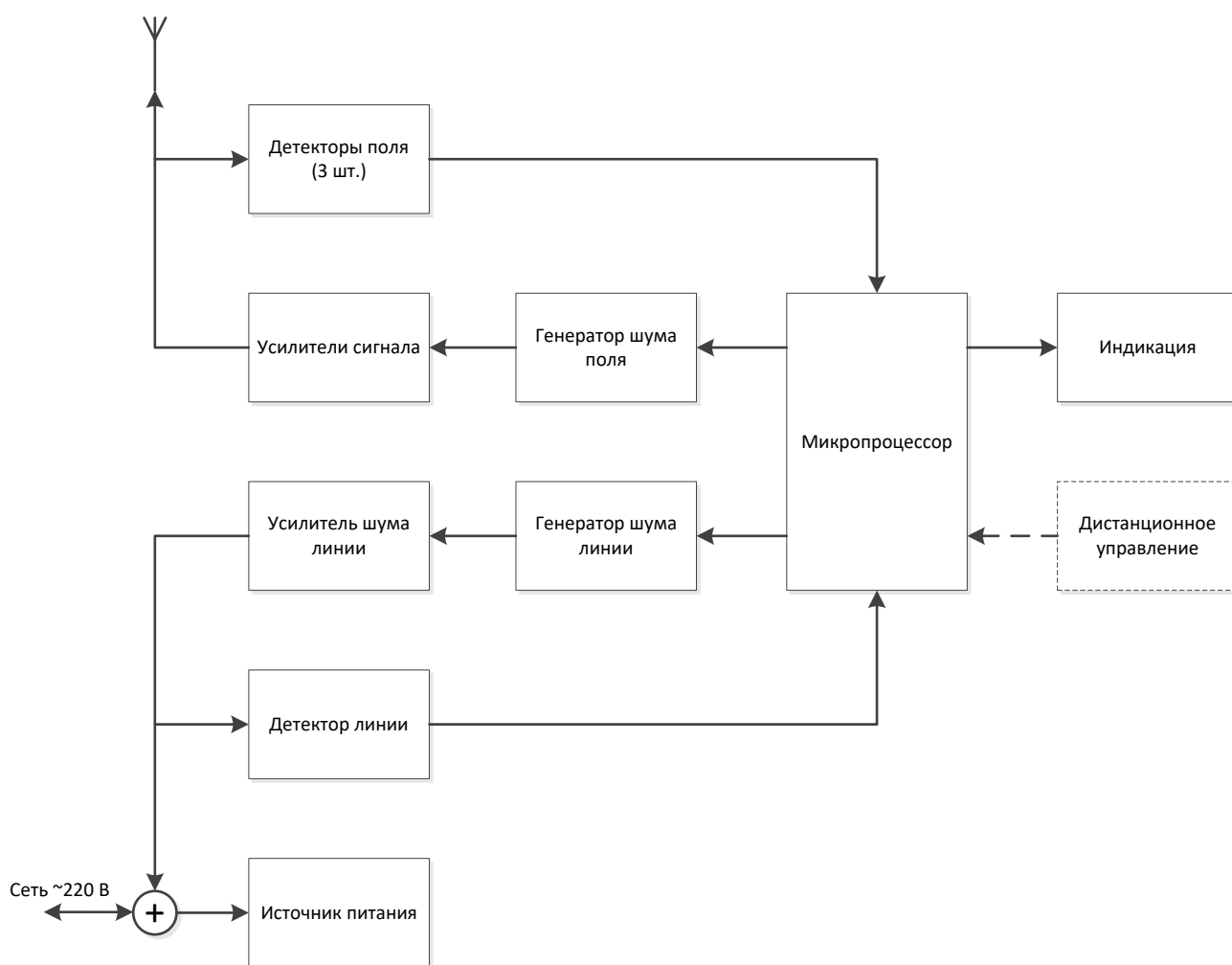
Рисунок 1 – Функциональная схема
