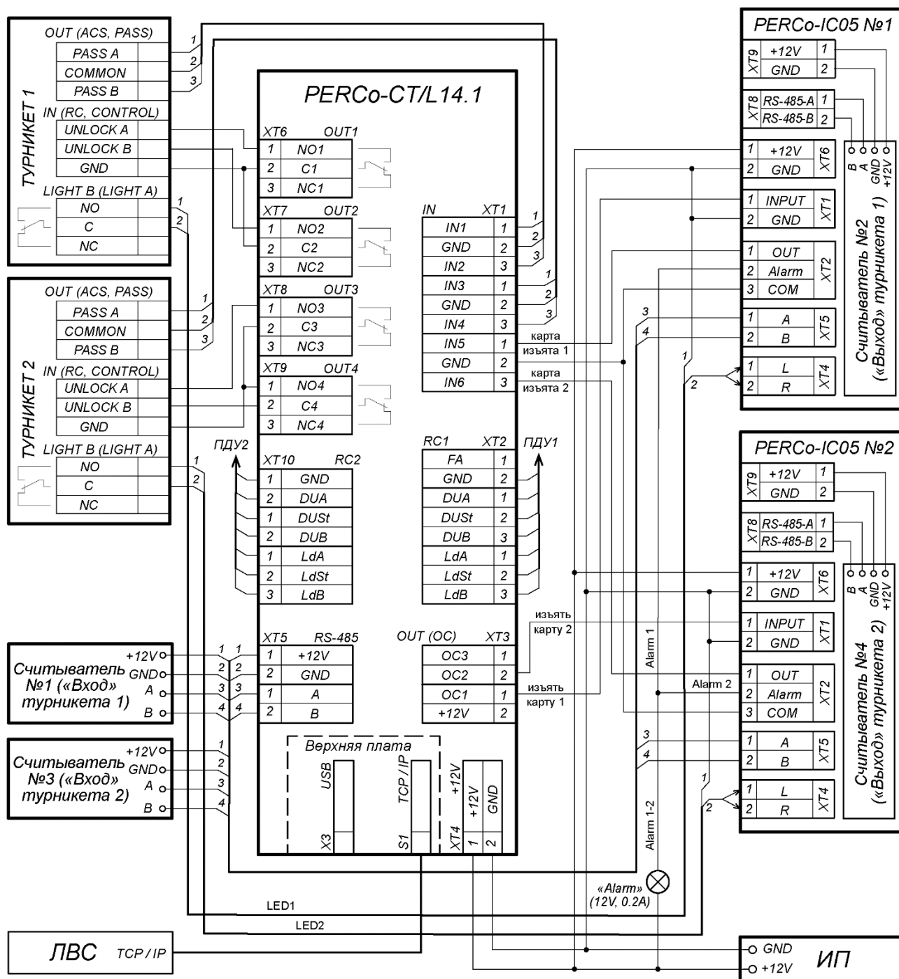
Рисунок 16. Схема подключения двух турникетов с картоприемниками PERCo-IC05
