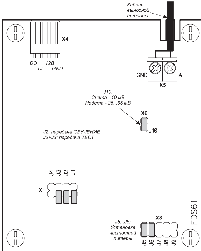
Рис. 2. Монтажная схема передатчика
